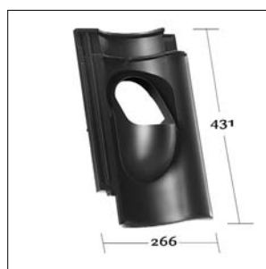
KE 0309 H 14 Hohlfalzziegel
