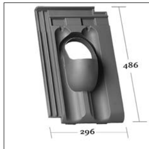
KE 0315 DS 10 Nibra
