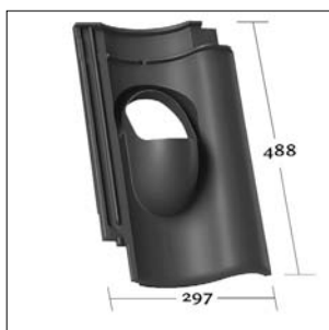
KE 0298 H 10 Hohlfalzziegel
